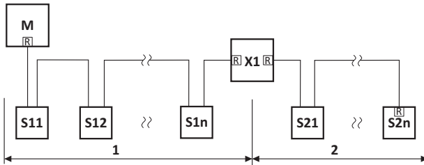
Abb. 4: Anschlussbeispiel: PROFIBUS-Netzwerk mit 2 Segmenten
