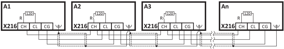
Abb. 2: Anschlussbeispiel: CANopen-Netzwerk
